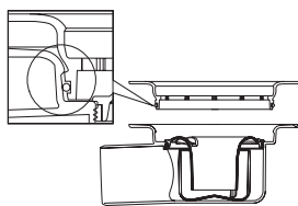
Anillos de elevación Anillo de sujeción automático. Disponible en las siguientes medidas para desagües 150: 13, 25, 50 y 100 mm. También está disponible uno flexible que facilita una elevación de 35-107 mm. Para los desagües 130 están disponibles en medidas de 13 y 25 mm: 13, 25, 50 and 100 and also a flexible ring that provides an extension of 35-107 mm. 13 and 25 mm rings are available for the 130 gully models.
