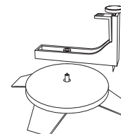
Cuchilla de Purus RSK 711 35 73 Ø80 Purus knife RSK 711 36 05 Ø130 RSK 711 35 94 Ø150 RSK 711 35 97 Ø220
