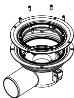
Anillos de elevación Anillo de sujeción atornillado serie S: 13 mm RSK 712 95 03 25 mm RSK 712 95 04 35 mm RSK 712 95 05 Extension rings Screwed clamping ring S-series: 13 mm RSK 712 95 03 25 mm RSK 712 95 04 35 mm RSK 712 95 05
