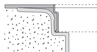
Anillos de resina Se utilizan sin el anillo de sujeción automático RSK 713 84 01 para desagüe 130 RSK 713 38 95 para desagüe 150 RSK 713 38 96 para desagüe 220 Resin rings Use without automatic clamping ring RSK 713 84 01 for 130 gully RSK 713 38 95 for 150 gully RSK 713 38 96 for 220 gully
